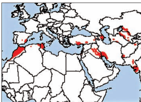
Figura 1 - Areale mondiale di nidificazione dell'Anatra marmorizzata (carta tratta da BirdLife International, 2004b).
