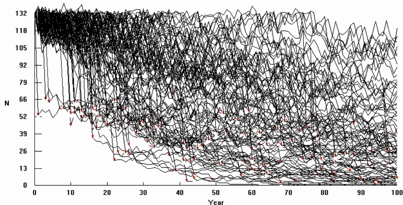
Fig. 1 - Trend di una ipotetica popolazione di 40 coppie con produttività pari a 0,97 giovani per coppia (vedi testo): probabilità di estinzione P \sim 0,17 in 100 anni.
